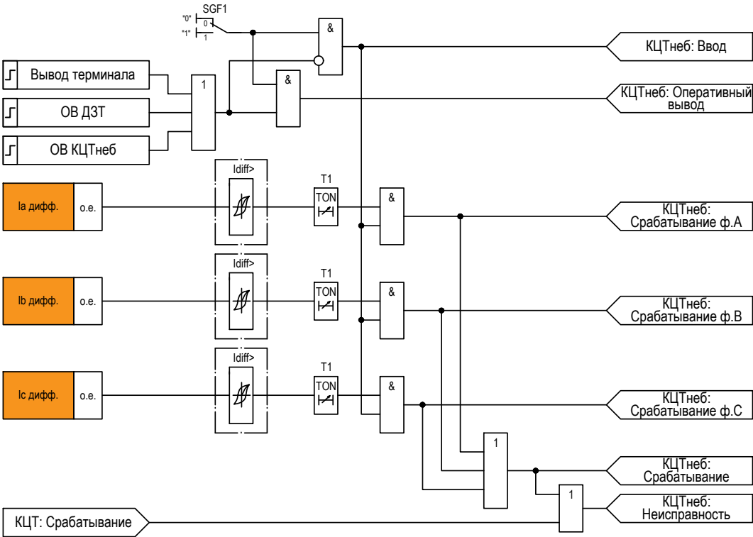
Рисунок 2.9 – Функциональная схема логики КЦТнеб
